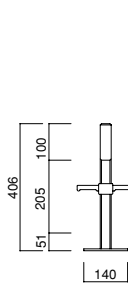
棒ジャッキ A-75T (A45)
