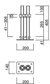
ダブルジャッキ A-752W (A44)
