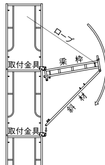
2) -2 上層にてロープを支持し、下層で斜材をガイドし、下の取付金具へ取付ける。
