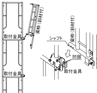
2) -1 上の取付金具の凹部へ梁枳のシャフトを掛ける。
