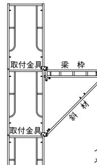
2) -3 上下の取付金具へ梁枳と斜材をボルトで固定する。
