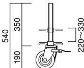
ジャッキ付キャスター A-728J...7.4kg
