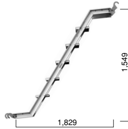
足場付階段枠 K-3615SA...14.0kg 幅420 (アルミ)
