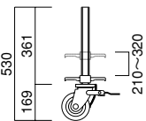
ジャッキ付キャスター A-726J...5.7kg
