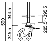
ジャッキ付キャスター A-728J...7.4kg
