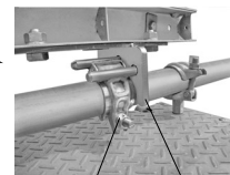
アサガオクランプ
