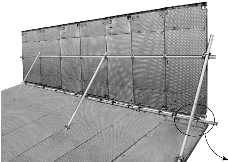
アサガオ金具 BSP-AK...1.7kg
