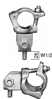
ボルト付単自在クランプ BSP-C1F...0.88kg
