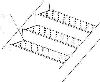
踏 板 TK-900ST 900×250×45
