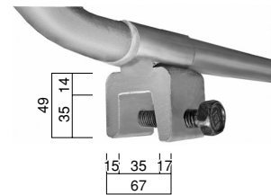
C型取付金具
