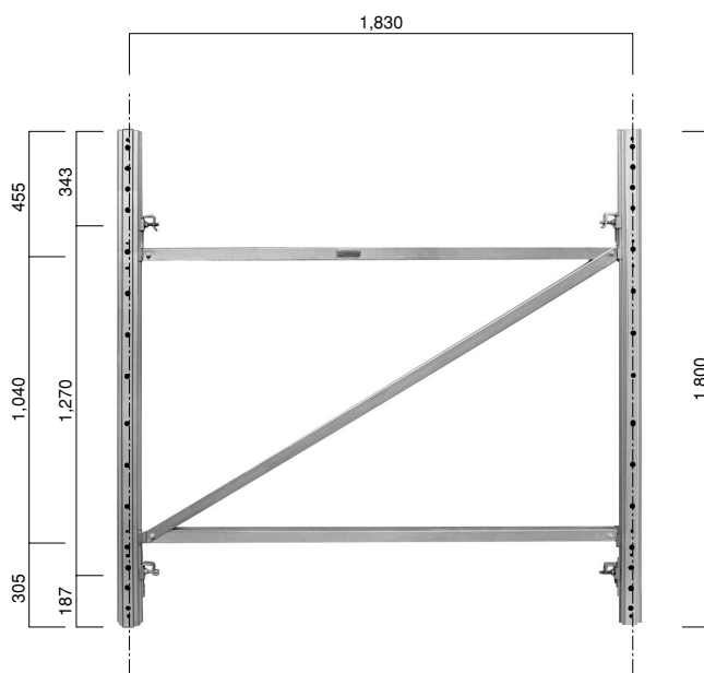
フレーム AL-F6×6…20.0kg (アルミ)
