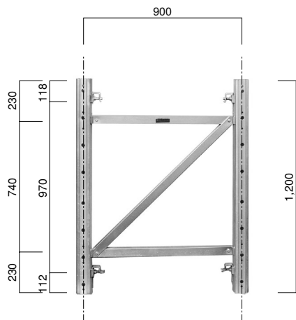
フレーム AL-F3×4…12.5kg (アルミ)
