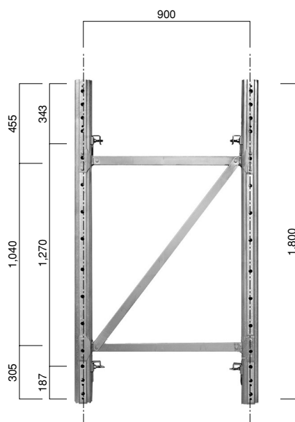
フレーム AL-F3×6…16.5kg (アルミ)
