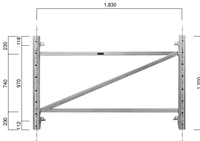
フレーム AL-F6×4…16.5kg (アルミ)
