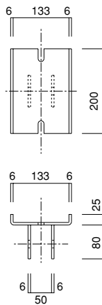
チルト大引受 AL-HP…2.50kg
