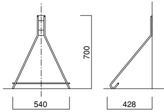
サポートスタンド AL-STD…1.75kg
