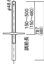
スクリュージャッキ AL-787J…6.70kg AL-580J (AL-580用) ( )内がAL-580J寸法
