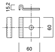
ジョーズクランプ AL-02D…0.13kg
