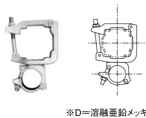
アルマクランプ KF-88D…1.00kg KF-88…1.00kg (自在)
