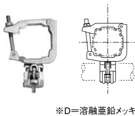
アルマクランプ KM-88D…1.00kg KM-88…1.00kg (直交)
