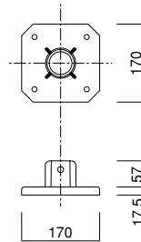
ベースプレート AL-BP…1.50kg (アルミ)
