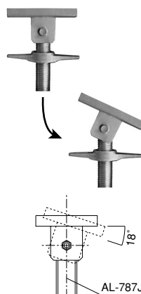
チルト大引受 AL-HP…2.50kg
