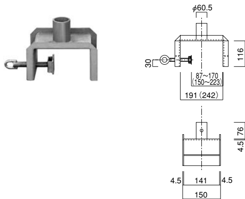
バルコニーHSクランプ AL-19D…4.60kg AL-24D…5.00kg ( )内がAL-24D寸法
