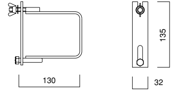
スタンドバンド AL-STB…0.70kg
