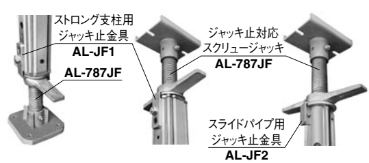
スクリージャッキ止め金具 AL-JF1…0.25kg AL-JF2…0.1kg AL-787JF…7.4kg
