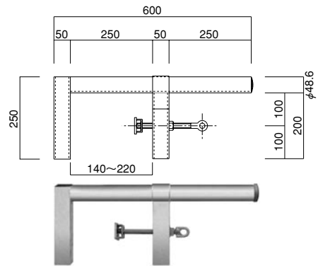
スクリージャッキ止め金具 AL-JF1…0.25kg AL-JF2…0.1kg AL-787JF…7.4kg
