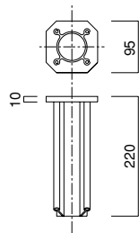
ベアリングキャップ AL-110…1.00kg
