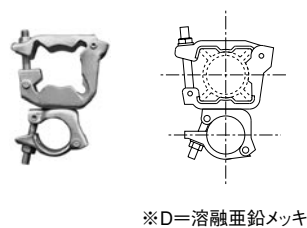
スライドパイプクランプ KF-67D…1.00kg KF-67…1.00kg (自在)
