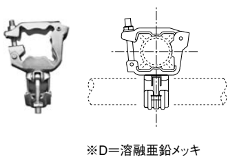
スライドパイプクランプ KM-67D…1.00kg KM-67…1.00kg (直交)
