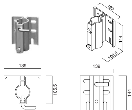
パイプソケット AL-48S…1.00kg (アルミ)
