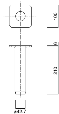
特殊ベアリングキャップ AL-H110…1.70kg
