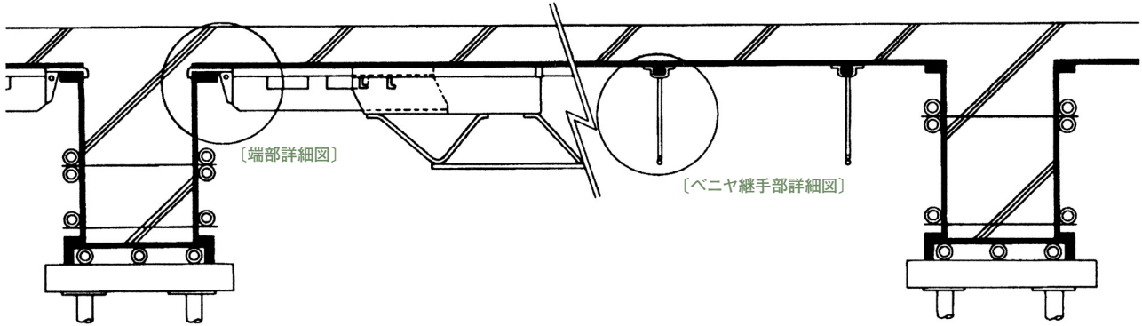
〔端部詳細図〕
