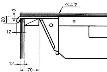
〔端部詳細図〕
